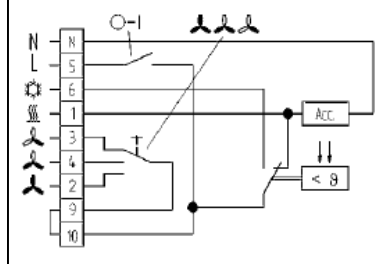
KLR-E 7009 kapcsolási rajza:
